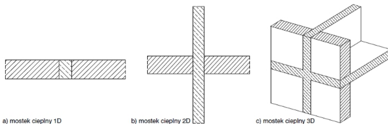
Rys. 1. Przykładowe mostki cieplne
