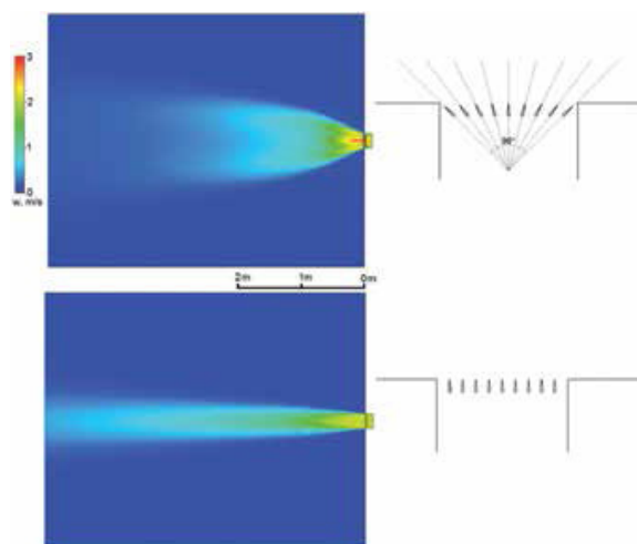
Rys. 3. Struga nawiewana z kratki w zależności od kąta ustawienia łopatek. Wymiary kratki to 225x125 mm, prędkość nawiewu 2 m/s.
