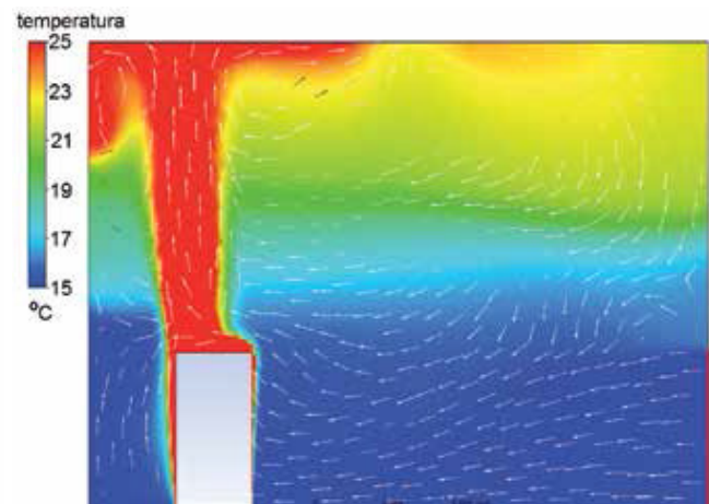
Rys. 5. Przepływ powietrza przy wentylacji wyporowej ze źródłem ciepła, w płaszczyźnie symetrii nawiewnika. Nawiewnik oznaczony jest czerwoną linią po lewej stronie.
