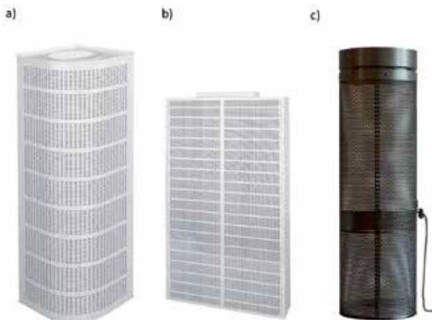
Fot. 6. Nawiewniki wyporowe: a) narożny [4], b) ścienny [4], c) przemysłowy do podwieszenia pod sufitem [6]
