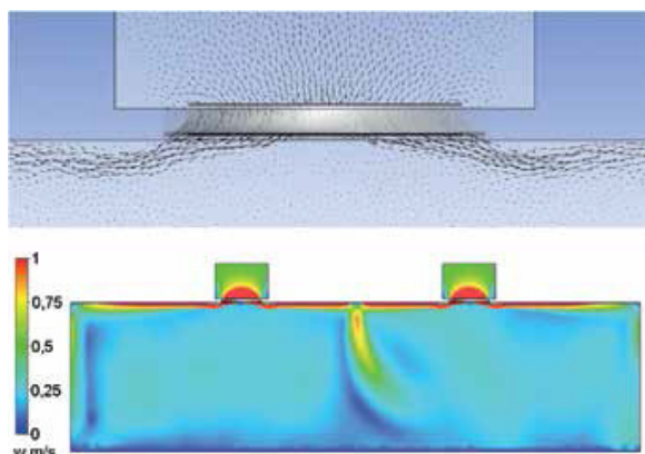
Rys. 1. Symulacja numeryczna wypływu powietrza z anemostatu (fot. 1a, c): a) wektorowy rozkład prędkości w pobliżu nawiewnika, b) rozkład prędkości na płaszczyźnie przecinającej dwa anemostaty umieszczone w pomieszczeniu. Odchylenie środkowej strugi spowodowane jest lokalizacją otworu wywiewnego po prawej stronie pomieszczenia.
