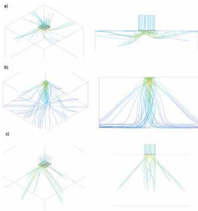
Rys. 2. Symulacja numeryczna wpływu powietrza z nawiewnika wirowego z ruchomymi łopatkami: a) struga przylegająca do sufitu (jak z anemostatu), b) struga zawirowana, c) strugi opadające bezpośrednio do strefy przebywania ludzi
